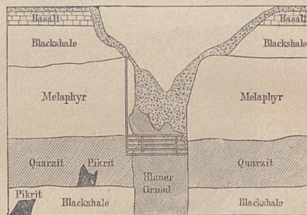
Fig. 1. Geologisches Profil der Kimberley-Mine.
