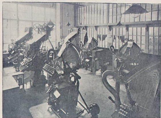
Setzmaschinenraum (cf. S. 36).
