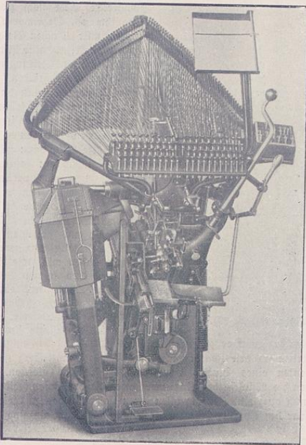
Typograph. Setzmaschine (cf. S. 30).
